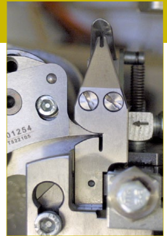
Stopfteil
