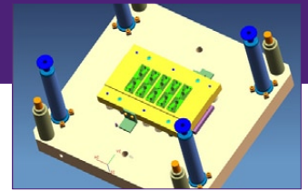
5-fach Schnitt Stempel
