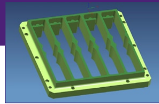
5-fach Matrize mit Aufhängeloch
