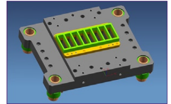
8-fach Schnitt Matrize
