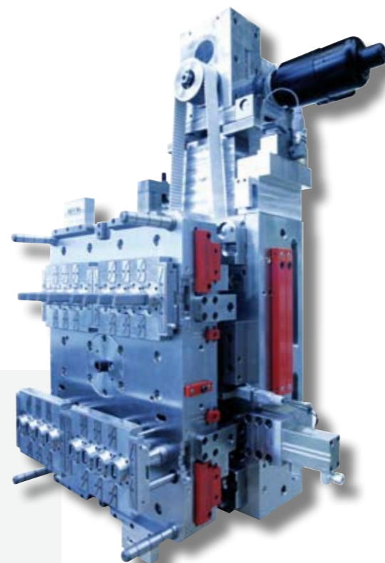
180° Drehplatte
