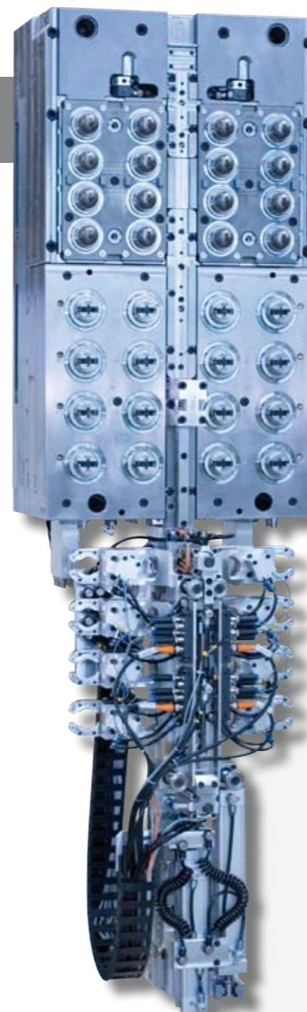
Werkzeuginternes Handling
